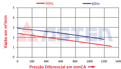
Curva Característica para Pressão
