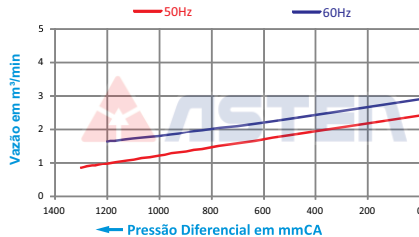
Curva Característica para Vácuo
