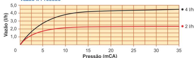
Agri Drip Auto-compensável Barb
